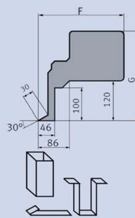
Abmessung Biegewanne HSBM SH
