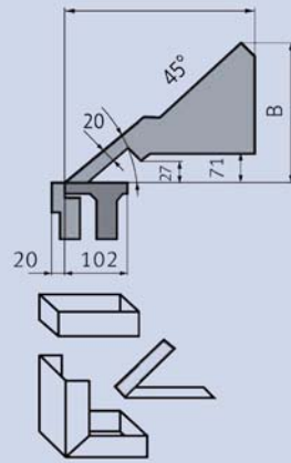
Abmessung Biegewanne HSBM S
