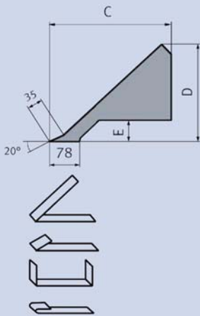
Abmessung Biegewanne HSBM
