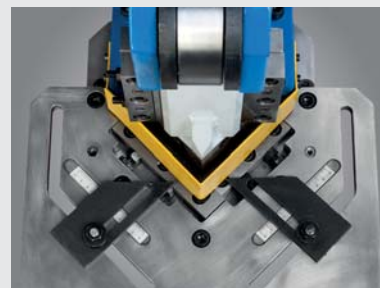
Skaleneinstellung
